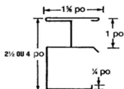
montant CH stud
