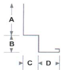
moulure MS moulding
