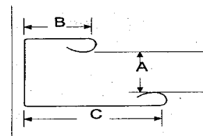
moulure US moulding
