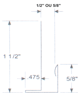
moulure MF moulding
